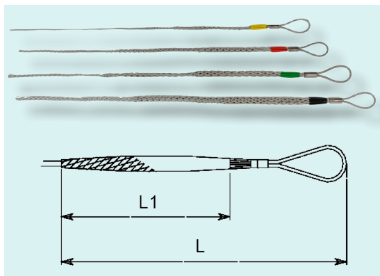
Головні затискачі «панчоха» для протягування проводів.
